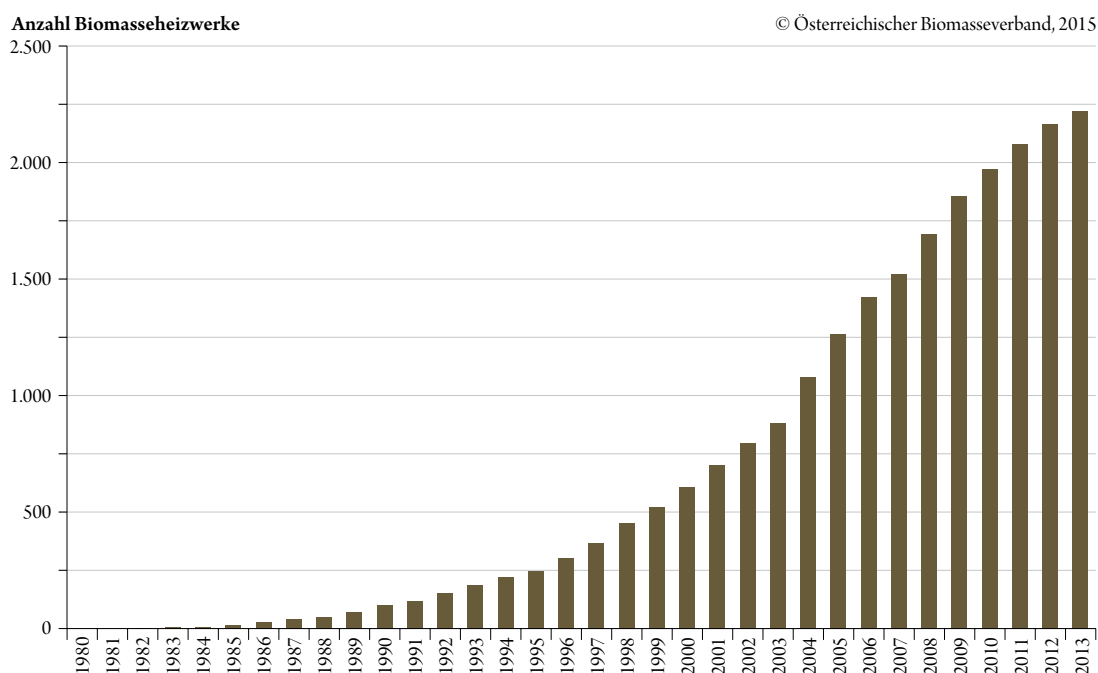
Entwicklung der Biomasseheizwerke in Österreich
